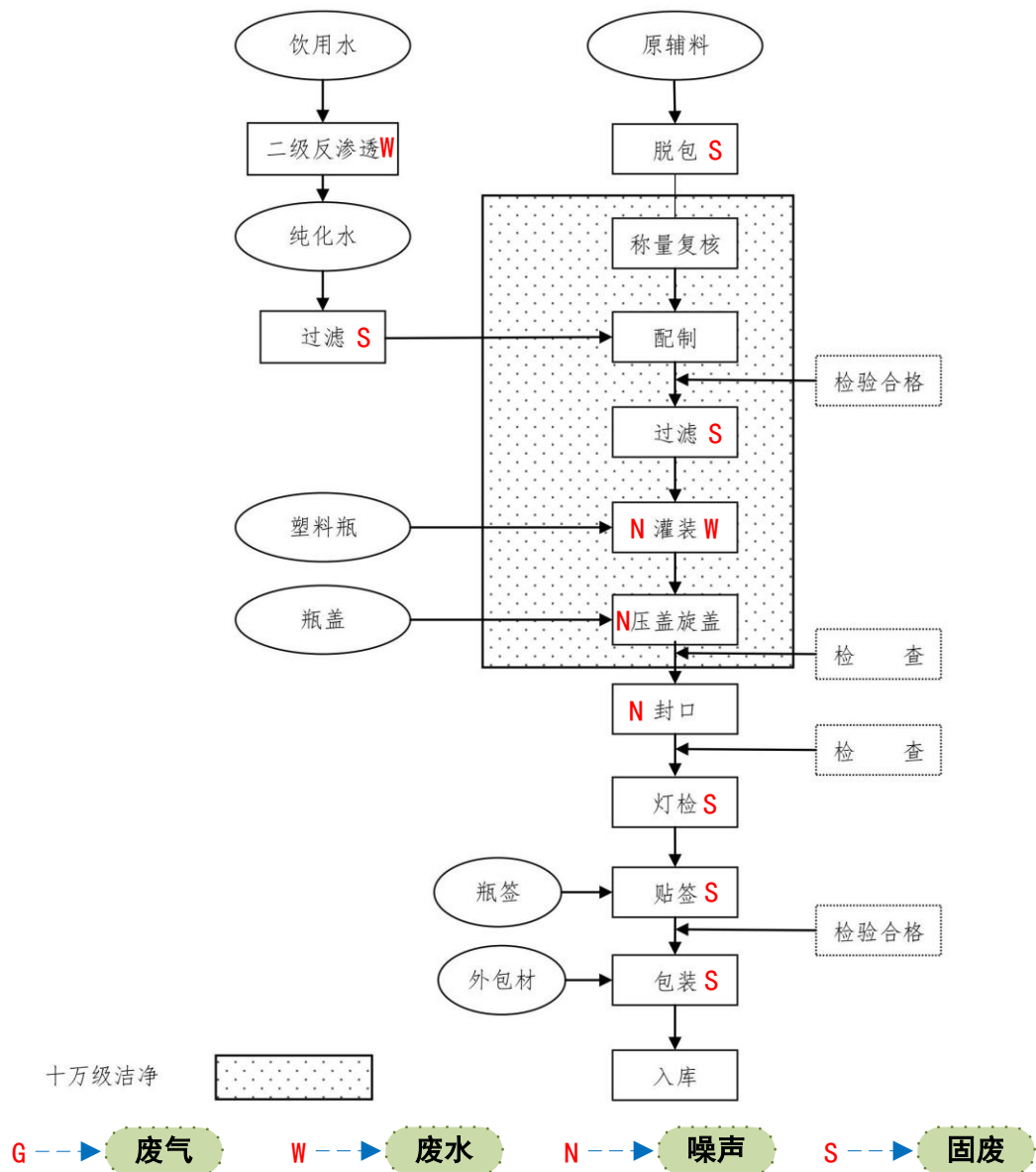
图 5-7 口服溶液剂/酞剂生产工艺流程及产污环节示意图
