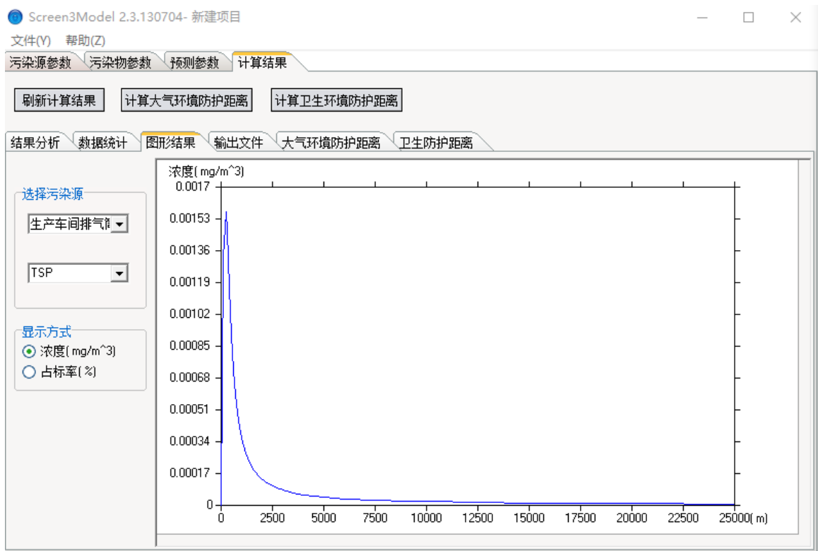
图 7-1 正常排放情况排气筒颗粒物排放浓度曲线
