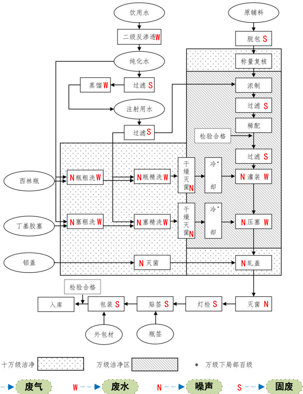
图 5-6 最终灭菌大容量非静脉/静脉注射剂生产工艺流程及产污环节示意图 生产工艺流程简述：
