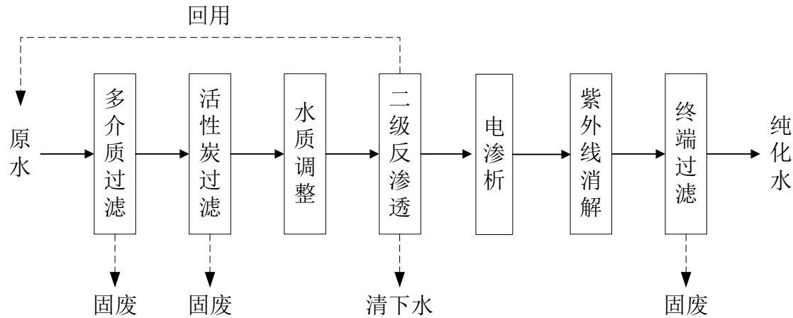
图 5-12 纯化水制备工艺流程及产污环节示意图
