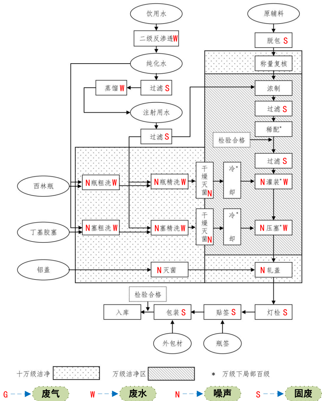
图 5-4 非最终灭菌大/小容量注射剂生产工艺流程及产污环节示意图
