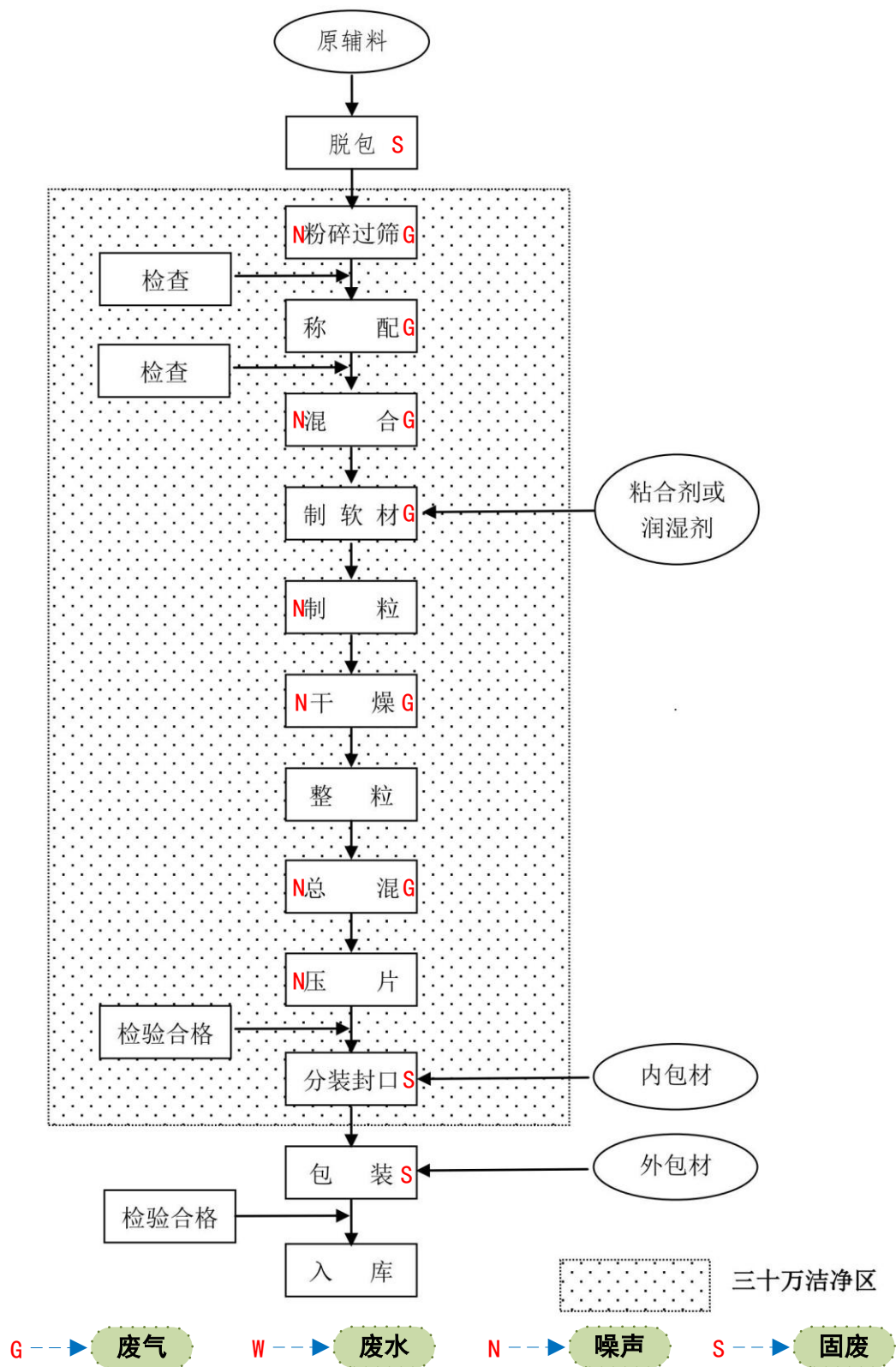
图 5-9 片剂生产工艺流程及产污环节示意图
