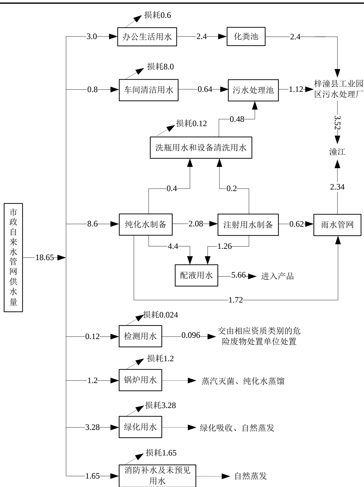
图 5-13 项目水量平衡图 (m³/d)
