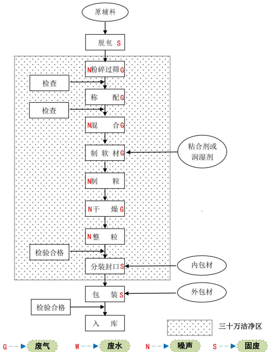
图 5-8 颗粒剂生产工艺流程及产污环节示意图
