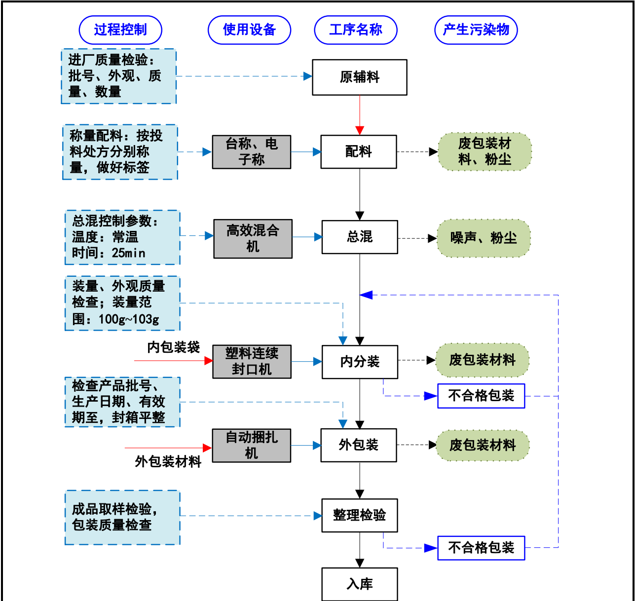
图 5-2 粉散剂生产工艺流程及产污环节示意图
