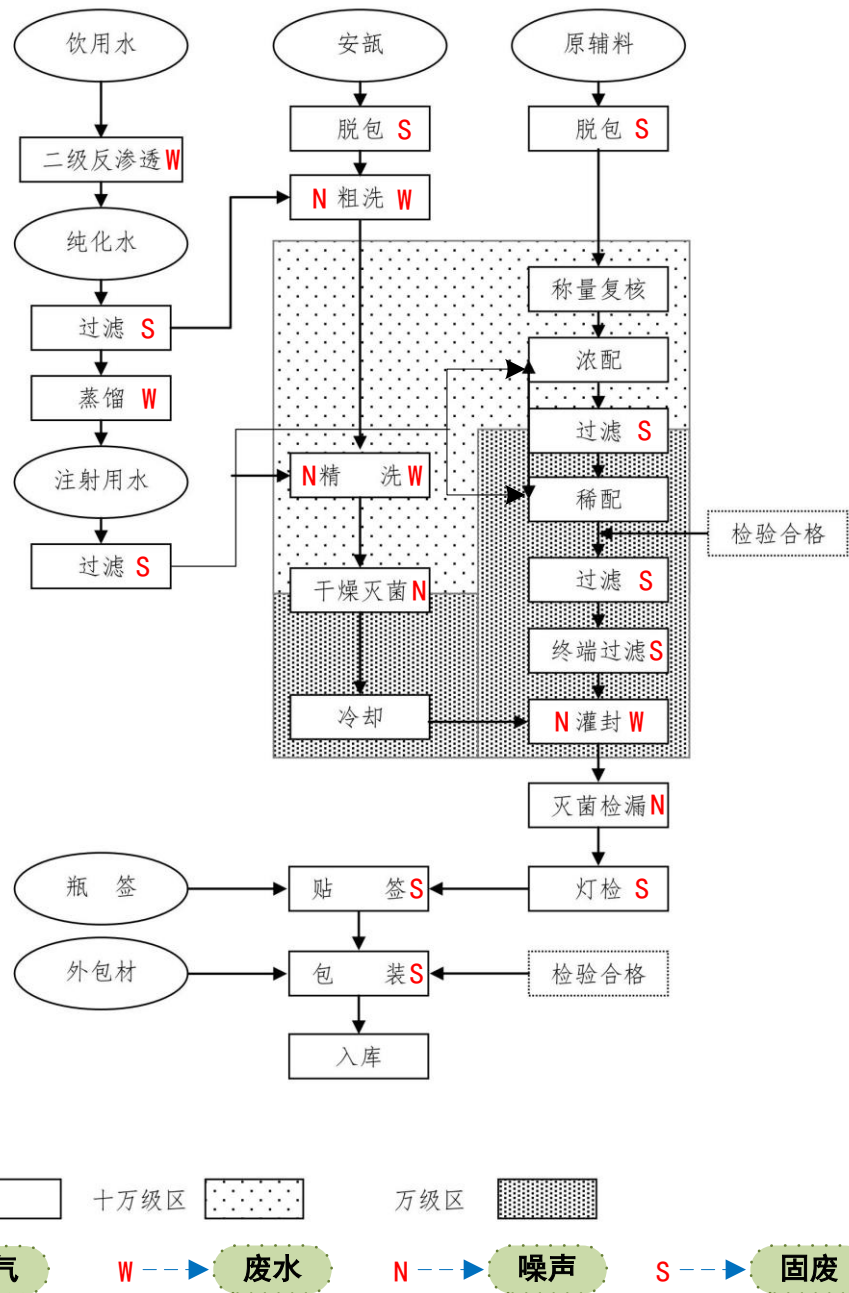
图 5-5 最终灭菌小容量注射剂生产工艺流程及产污环节示意图
