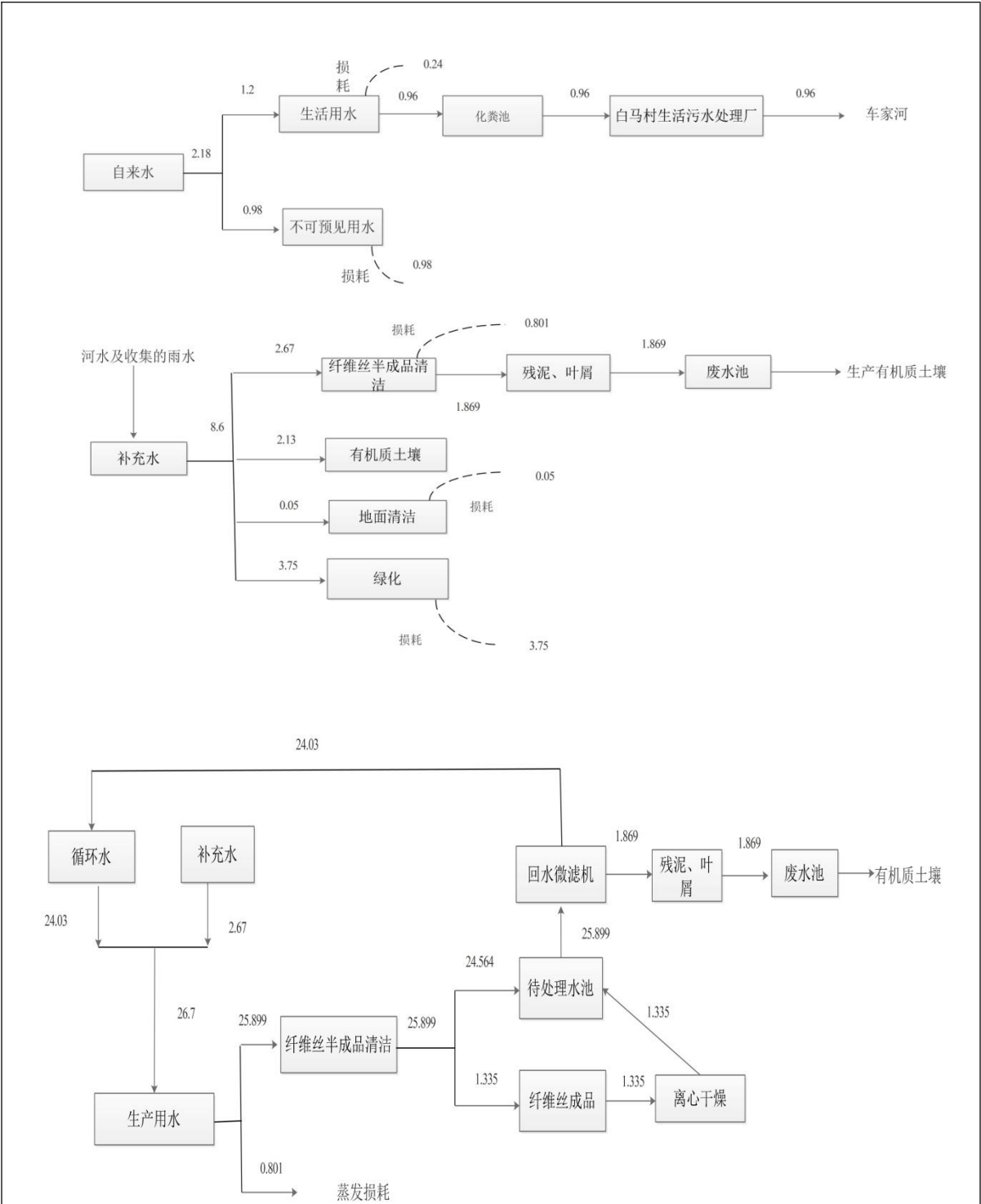
图 5-4 项目水平衡分析图（单位 m³/d）
