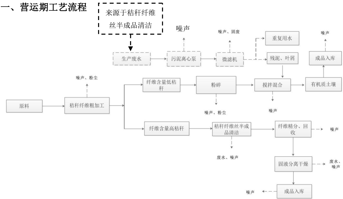
图 5-3 运营期工艺流程及产污位置图
