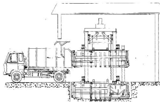
图 5-6 对接卸料图
