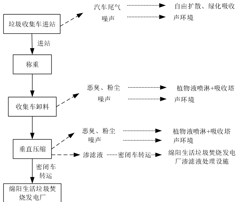
图 5-2 运营期工艺流程及产污环节图
