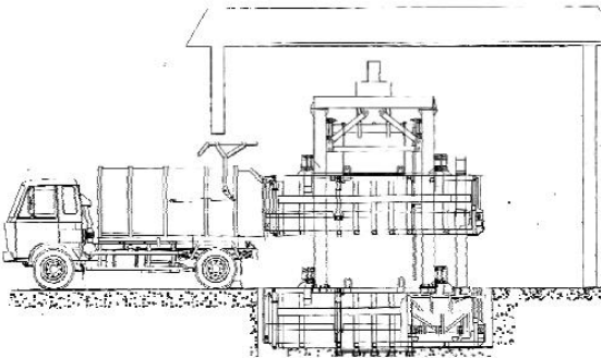
图 5-6 对接卸料图
