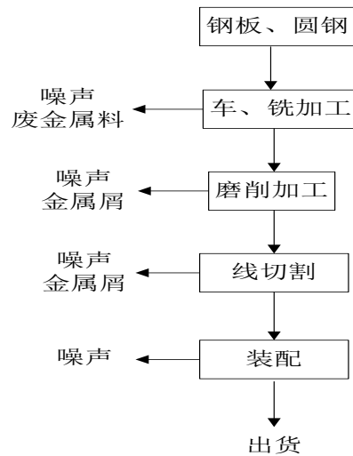
图 5-2 项目工艺流程及产污环节图
