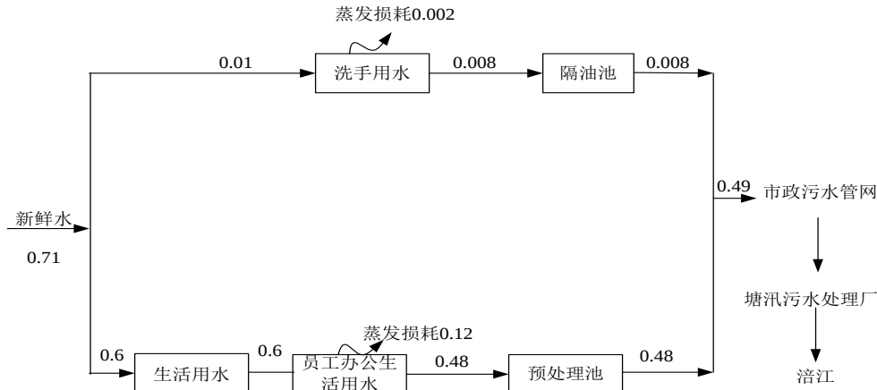
图 5-3 项目水平衡图 单位： \text{m}^3/\text{d}
