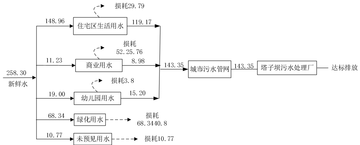
图 5-3 项目水平衡分析图（单位：m 3 /d）
