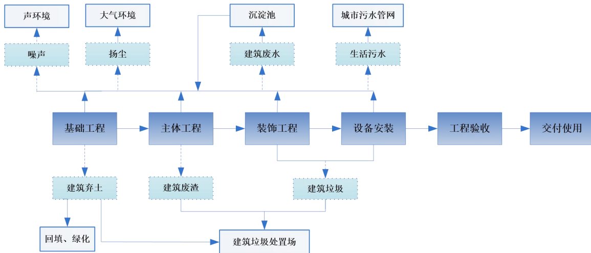
图 5-1 施工期工程工艺及产污位置图
