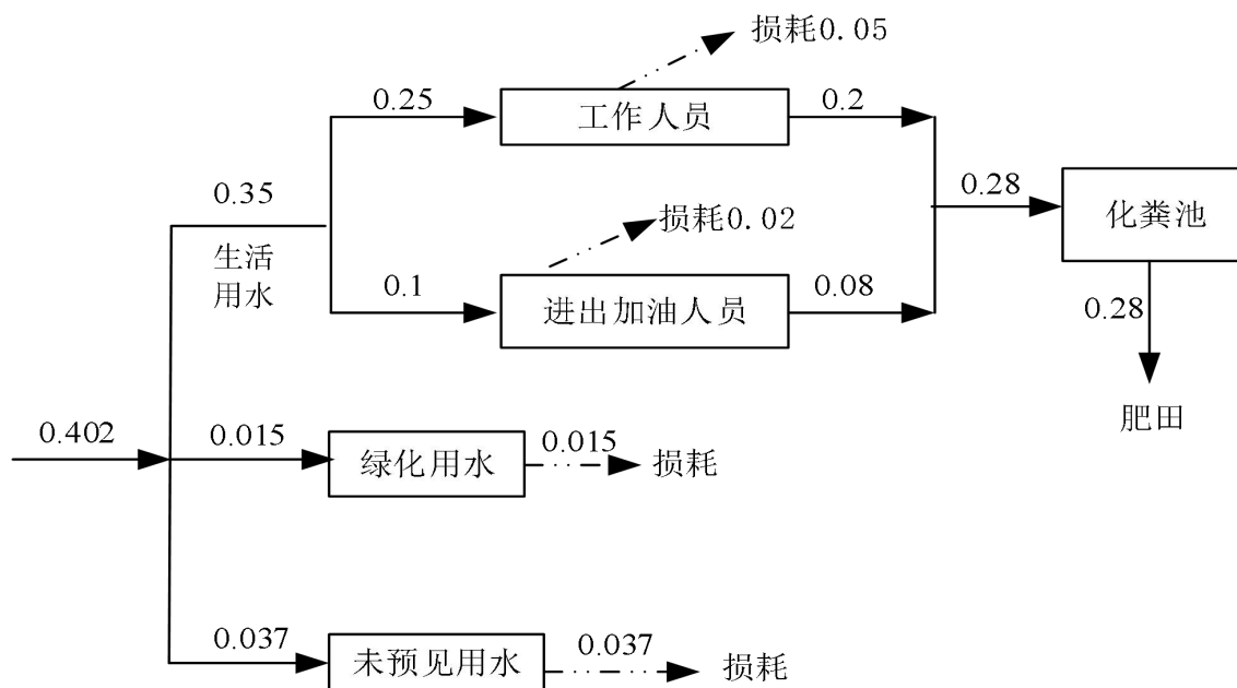
图 1 项目水平衡关系图 单位: \text{m}^3/\text{d}
