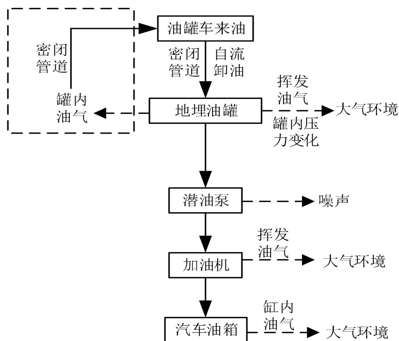
图 5-1 加油工艺流程及产污位置图
