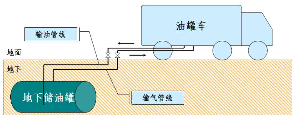
图 5-2 卸油油气回收系统示意图
