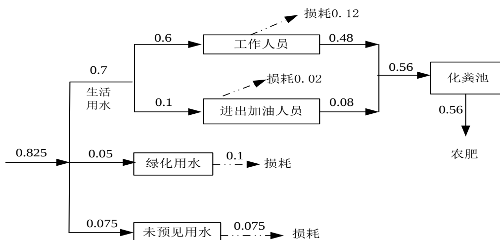
图 1-2 项目水平衡关系图 单位：m 3 /d
