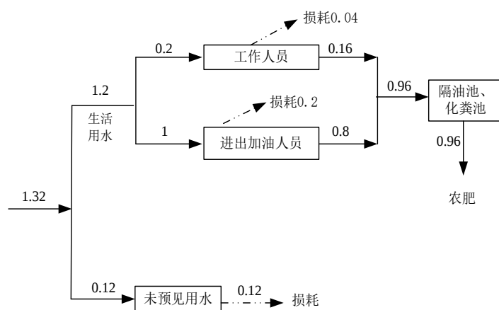
图 1-2 项目水平衡关系图 单位: m³/d
