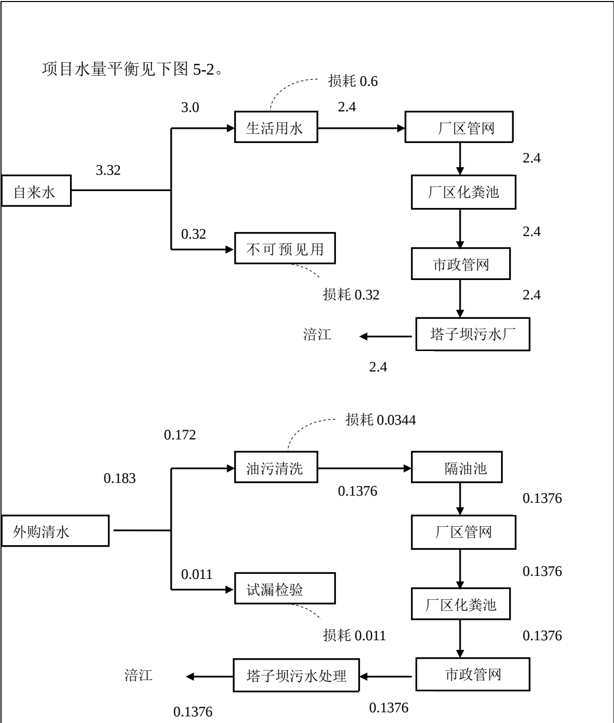
图 5-2 项目水平衡分析图（单位 m³/d）
